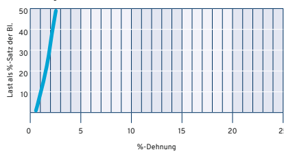
Dehnungskurve
